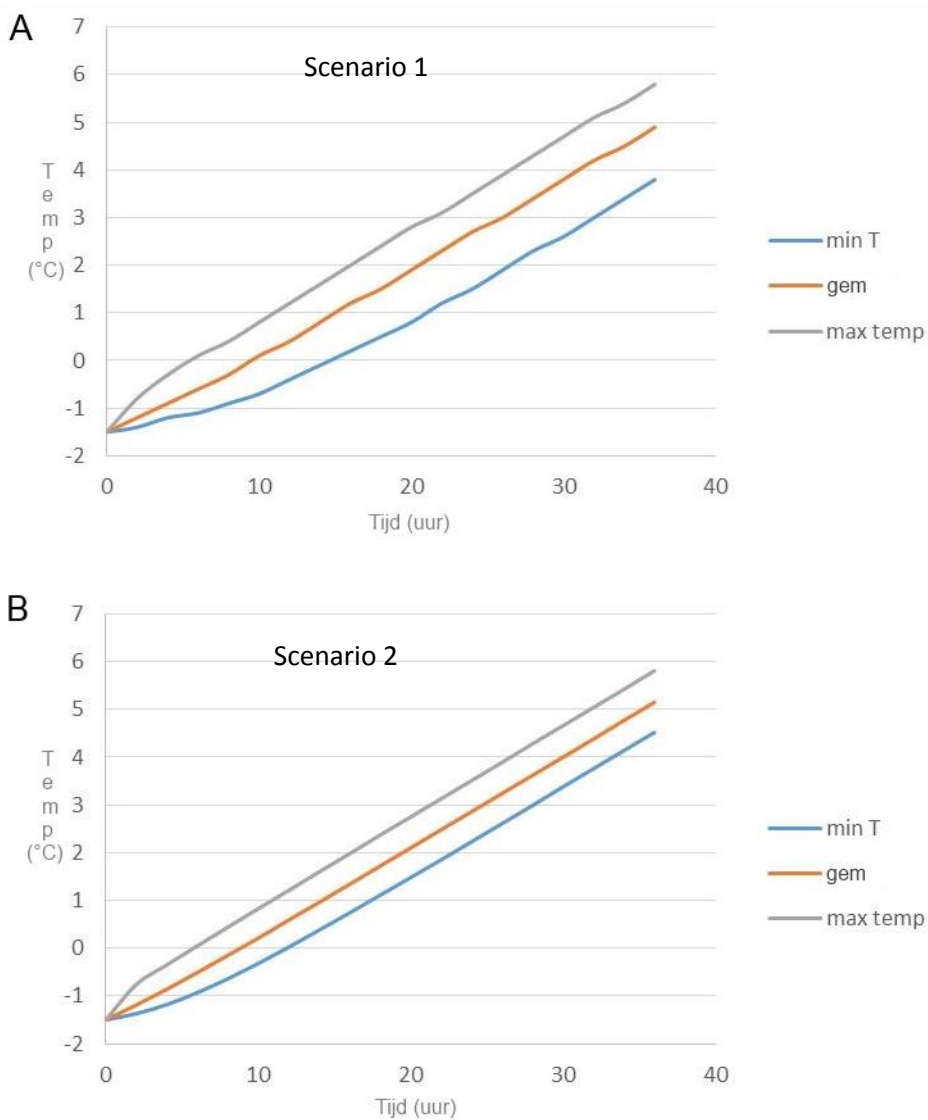
Figuur 2. Berekende temperatuursprofielen na 36 uur ontdooing in scenario 1 (A) en scenario 2 (B)
