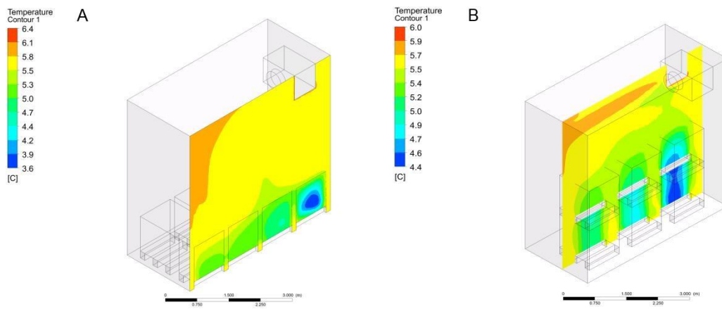
Figuur 2. Berekende temperatuursprofielen na 36 uur ontdooing in scenario 1 (A) en scenario 2 (B)
